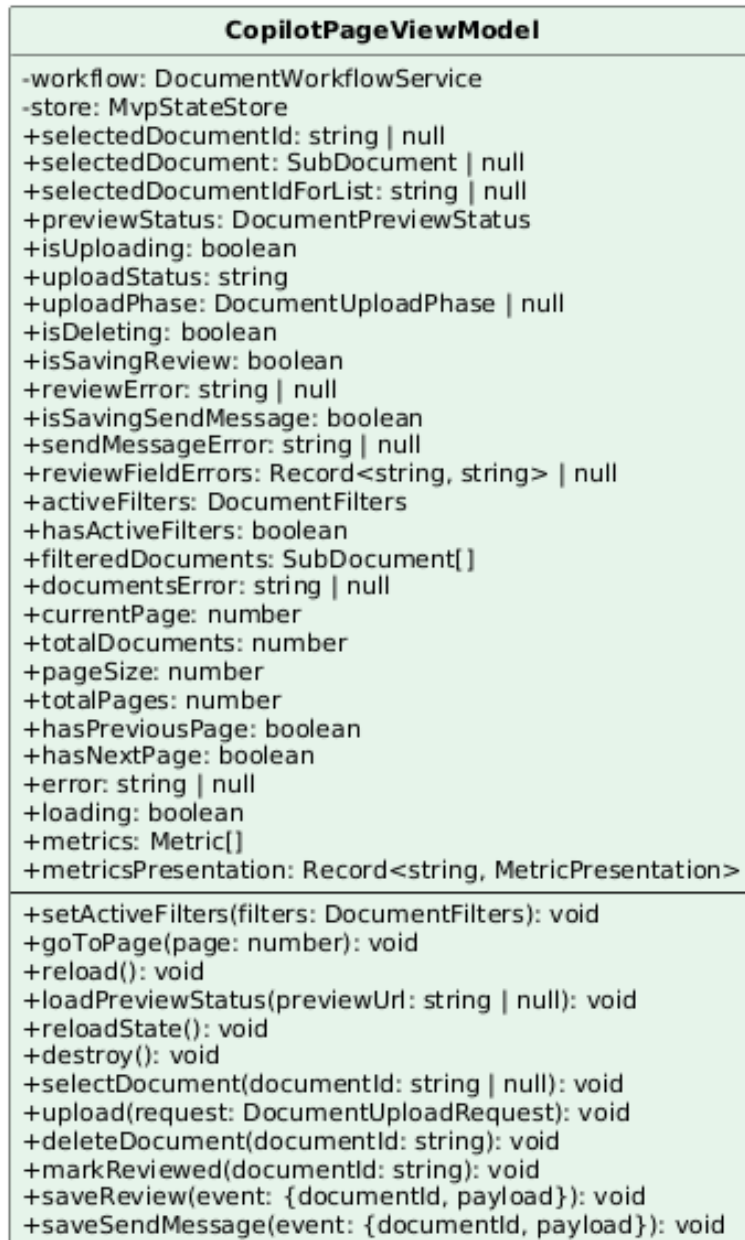
Figura 90: Classe: CopilotPageViewModel
